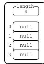
new int[4][] で生成される配列
